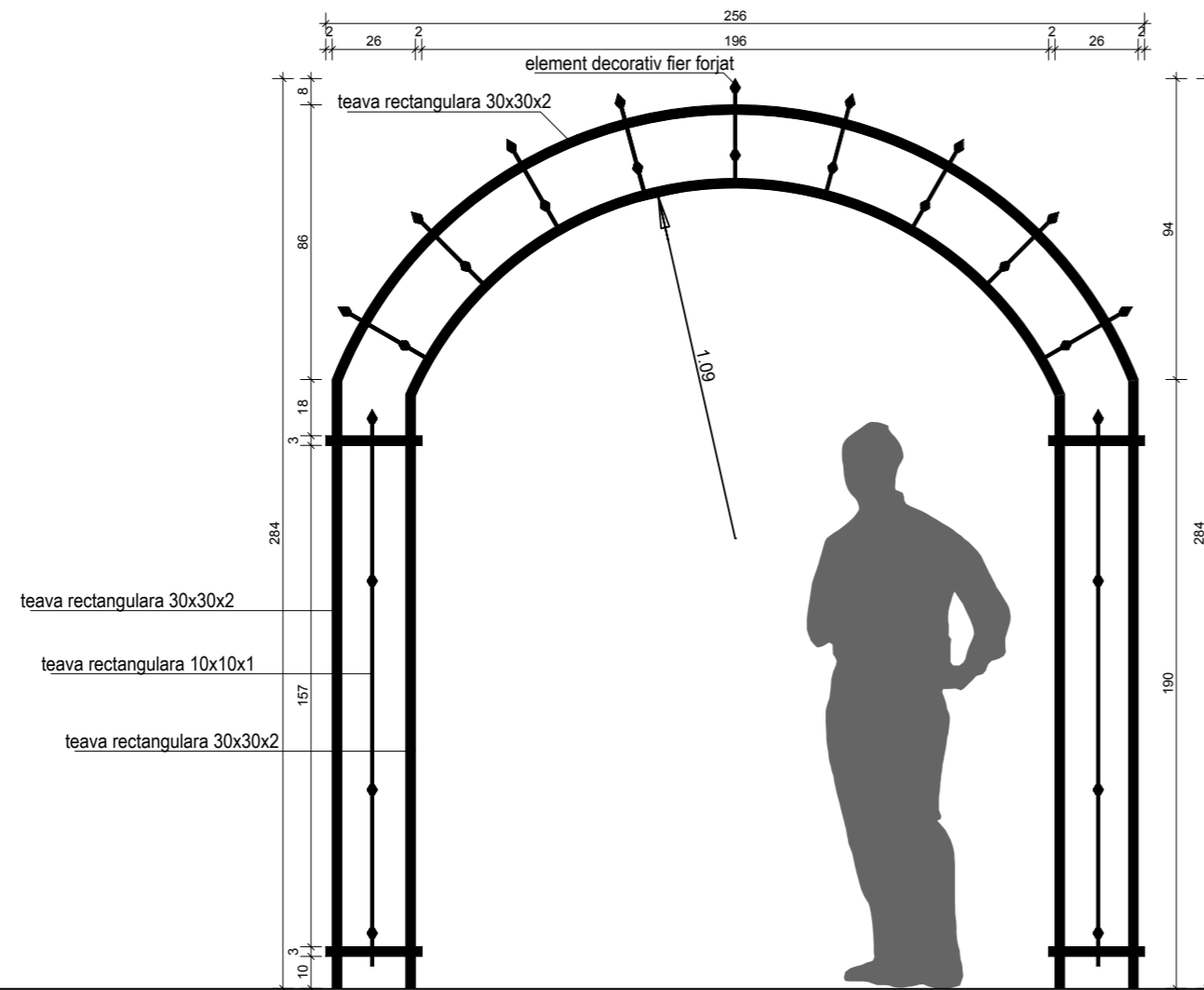
vedere frontala sc. 1:20
