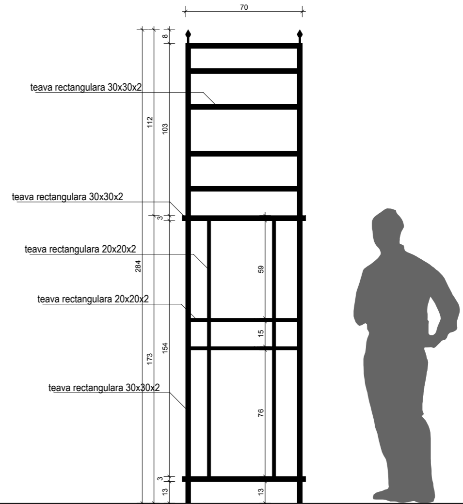
vedere laterala sc. 1:20
